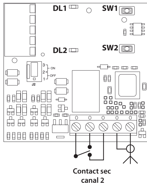
Récepteur BRAVO RPE 243 HG
